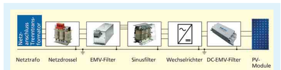
1 Filtermaßnahmen eines elektromagnetisch verträglichen dreiphasigen PV-Wechselrichters
