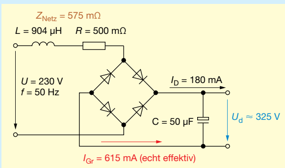
4 Schaltung und Parameter zu Bild 5
