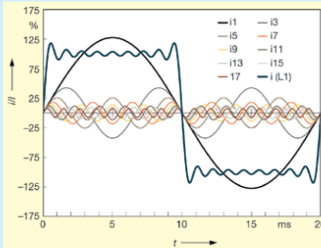
❷ Grafische Synthese eines Rechteckstroms (dick, dunkelblau) aus der Grundschwingung (schwarz) und den Oberschwingungen 3 bis 17
