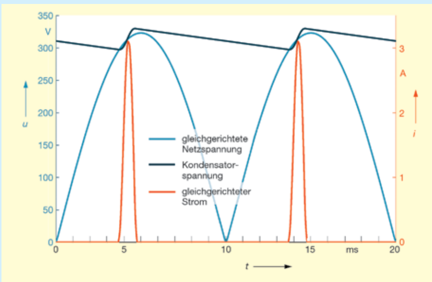
5 Sich rechnerisch ergebende Kurvenverläufe der Kondensatorspannung und des gleichgerichteten Netzstroms aus Bild 3
