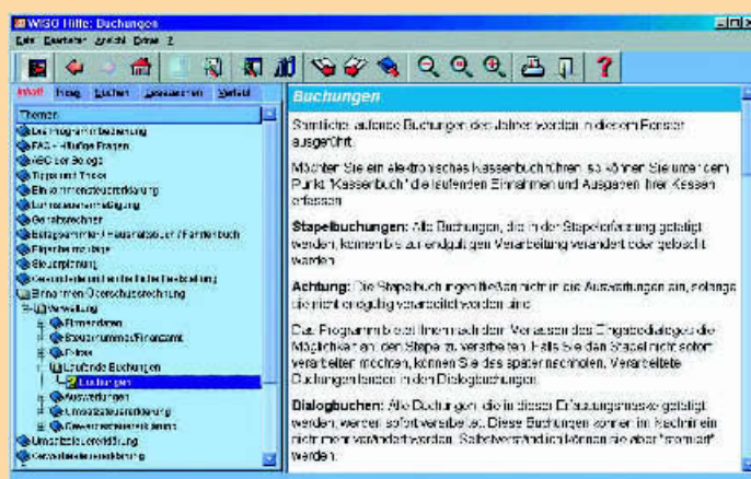
7 Interne Hilfe
