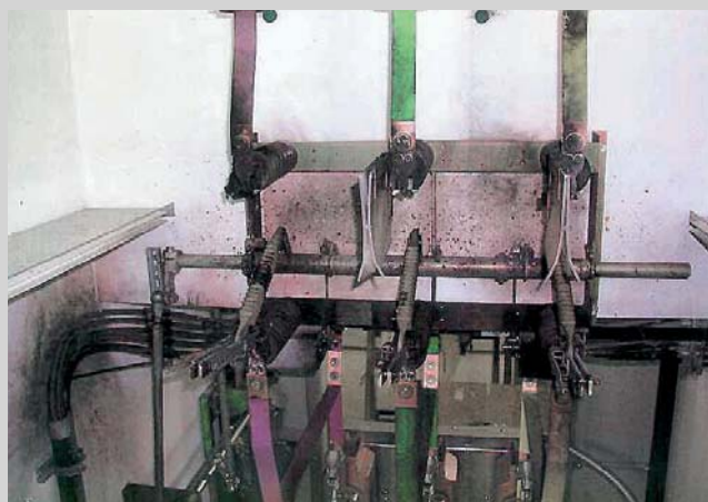
❶ 20-kV-Schaltfeld nach einem Lichtbogenunfall
