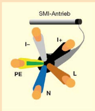
4 Anschluss über ein 5-adriges Kabel [1]
